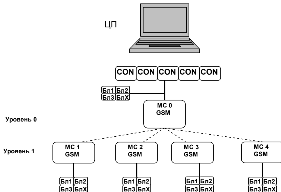
Рис 1. Структура системы MC – GSM
